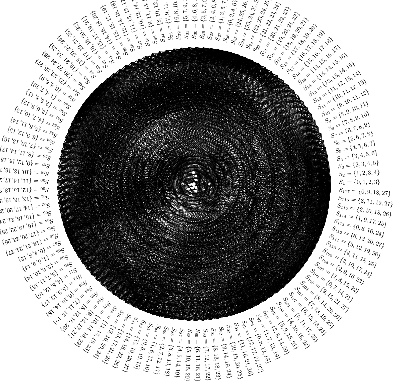
Graphe des progressions arithmétiques n = 7, k = 4
