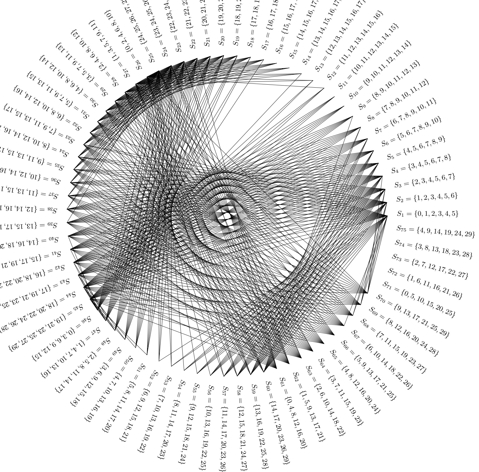
Graphe des progressions arithmétiques n = 5, k = 6
