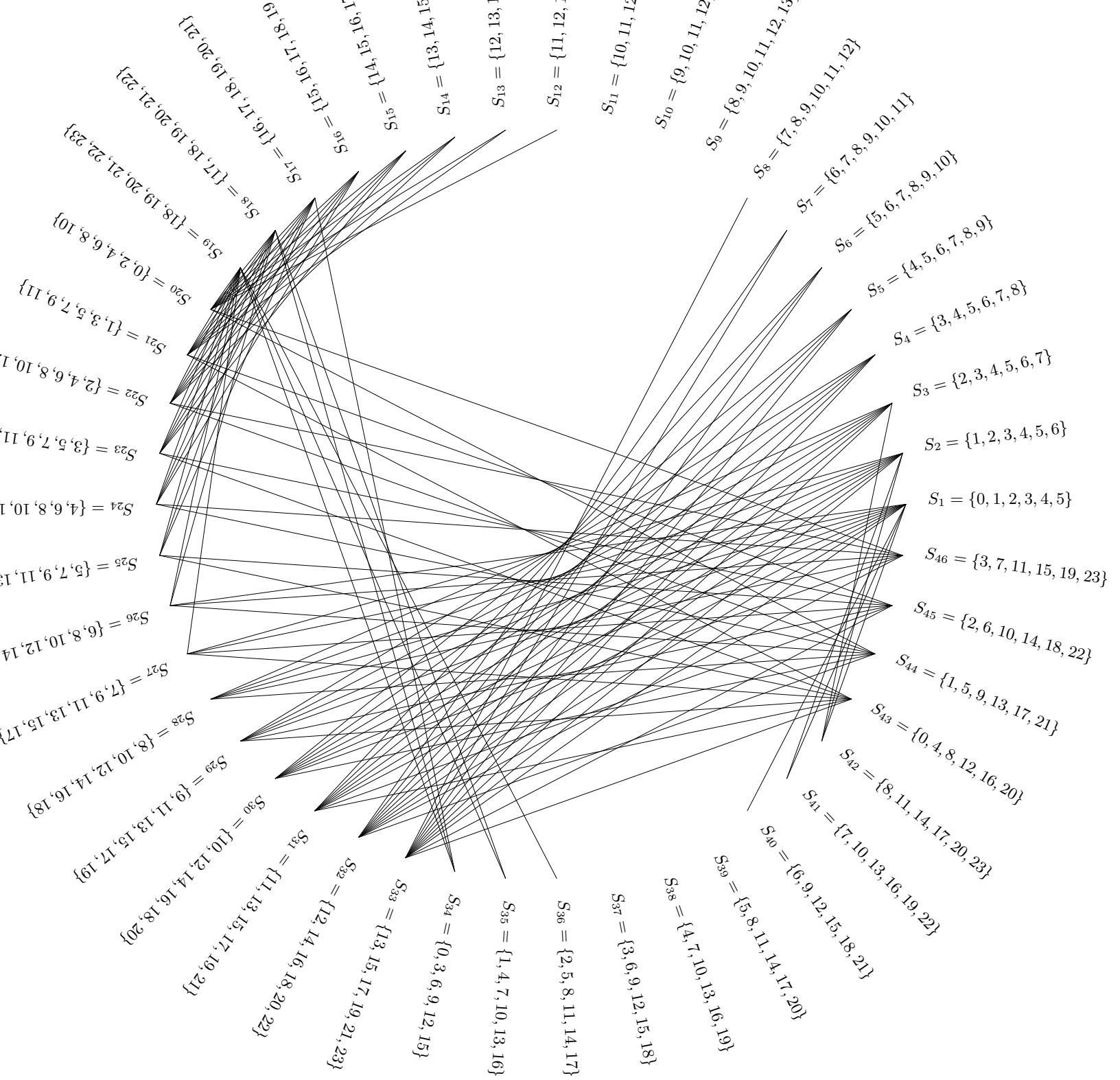
Graphe des progressions arithmétiques n = 4, k = 6
