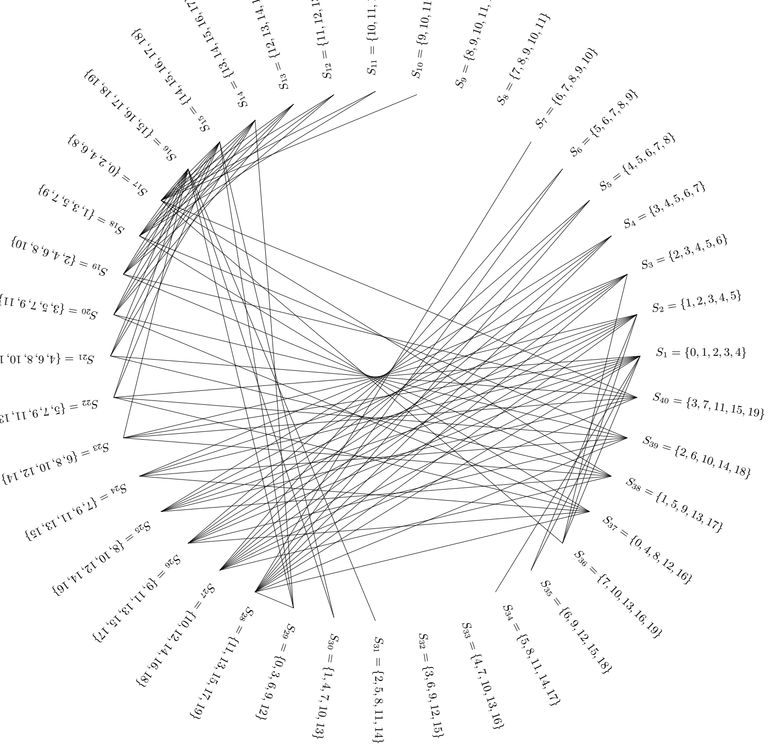
Graphe des progressions arithmétiques n = 4, k = 5
